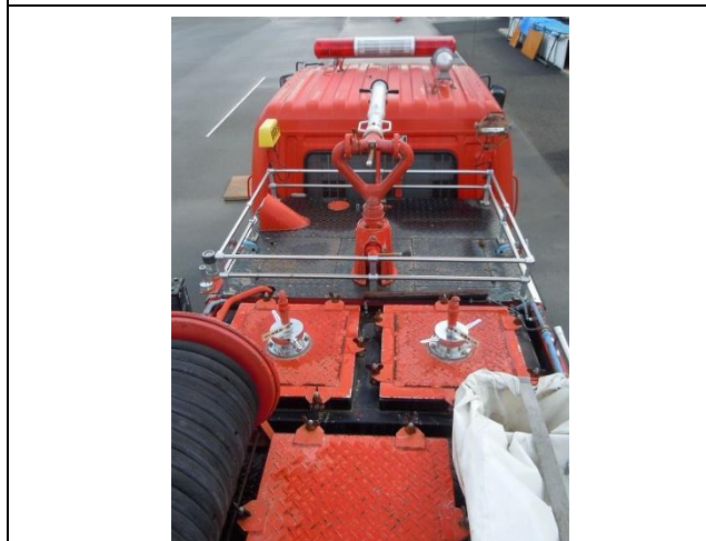
車体上部
